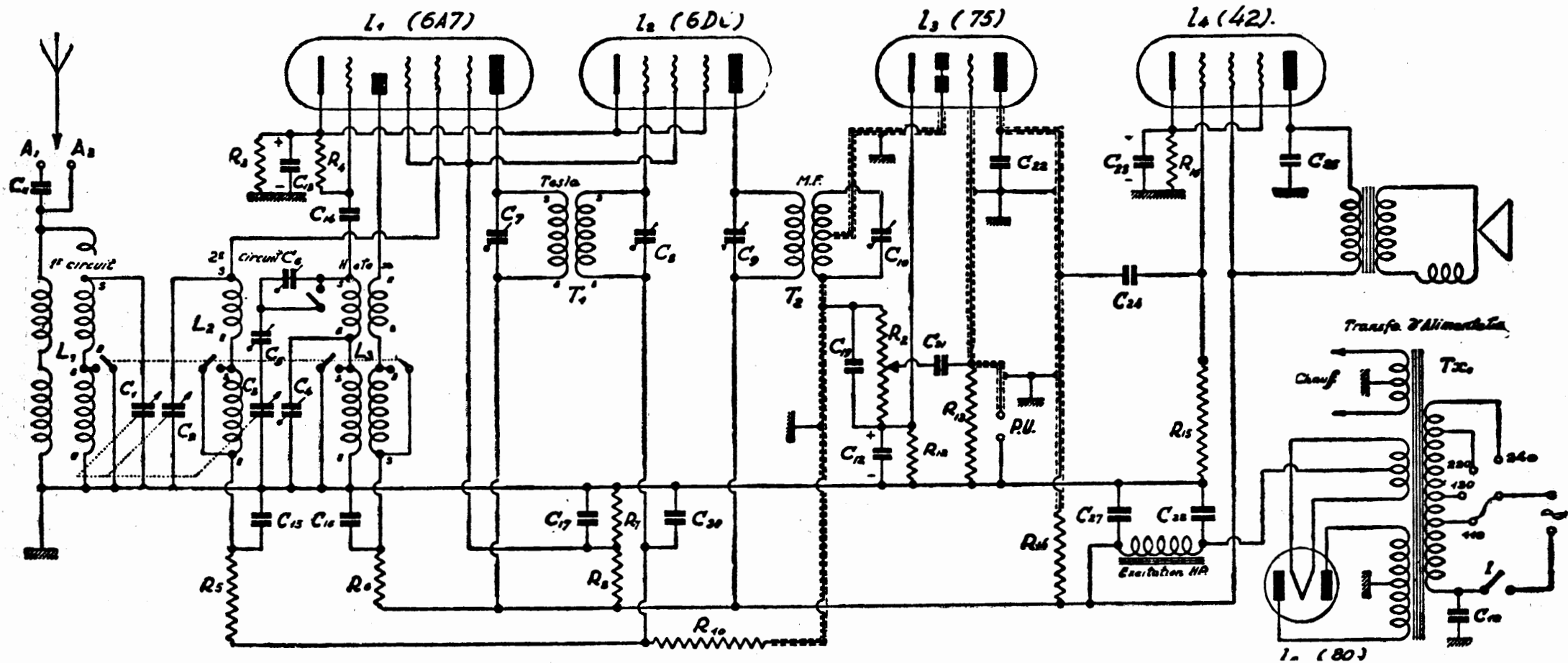
Schéma du superhétérodyne 3689 Radio LL.
