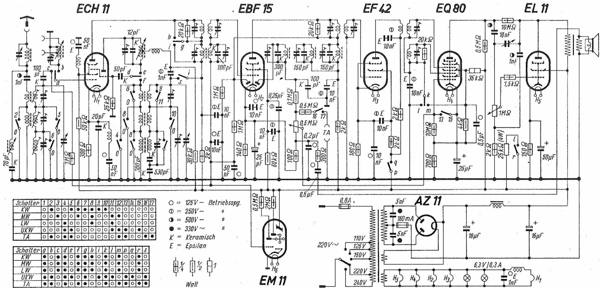
Bild 1. Service-Schaltbild des AM-FM-Superhets Lumophon WD 571 / US 2 mit Einzelteilwerten und Röhrenmeßdaten
